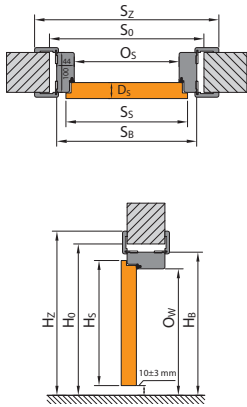
■ MINIMAX DOOR FRAME
